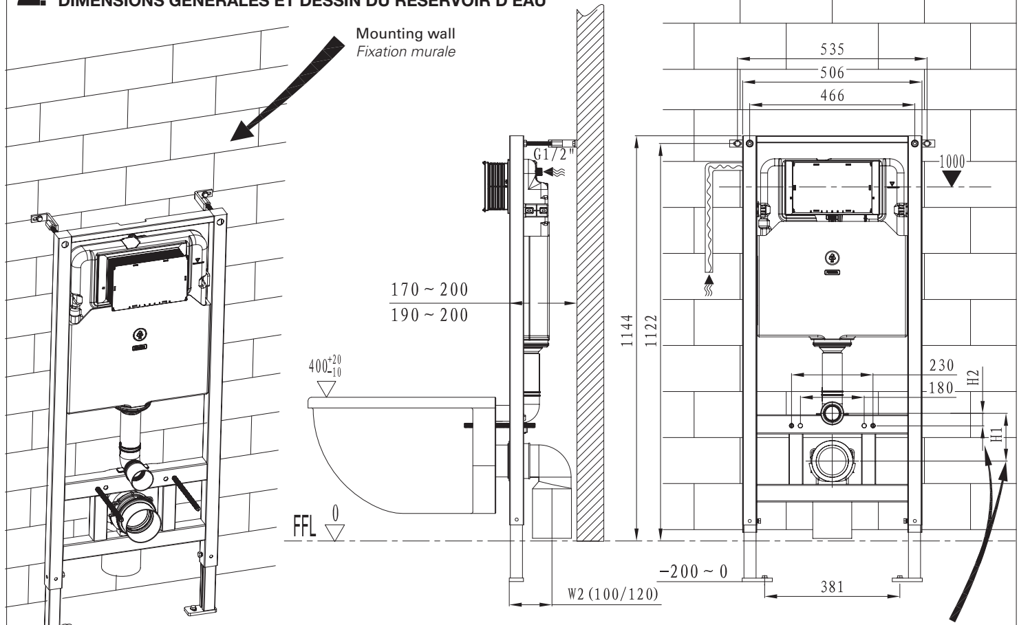
Dimensions of H1 and H2, depending on the parts used. Dimensions de H1 et H2, selon les pièces utilisées.
