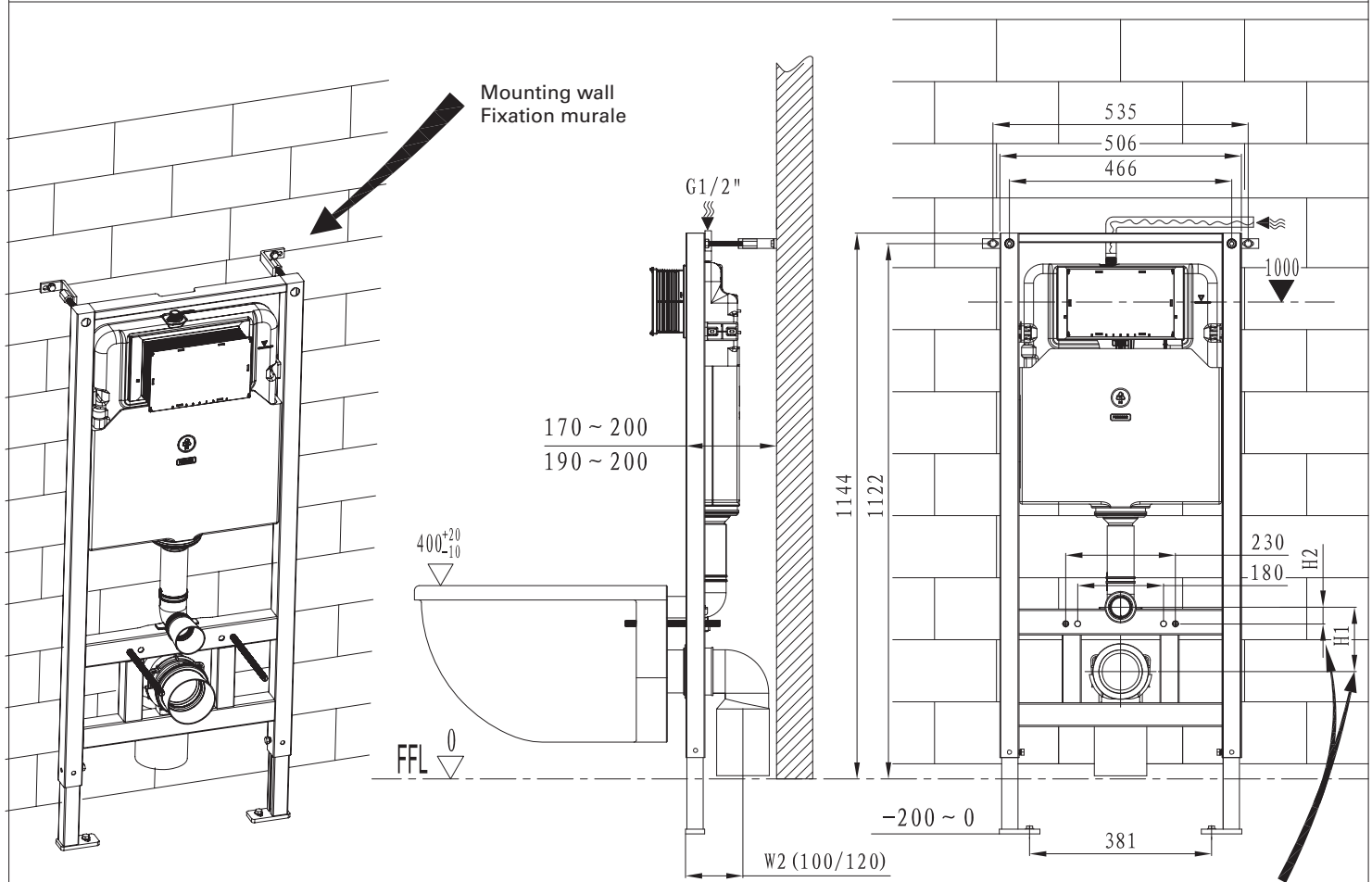
Dimensions of H1 and H2, depending on the parts used. Dimensions de H1 et H2, selon les pièces utilisées.
