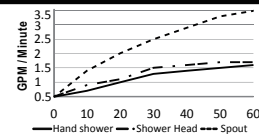
Flow rate chart Diagramme de débit
