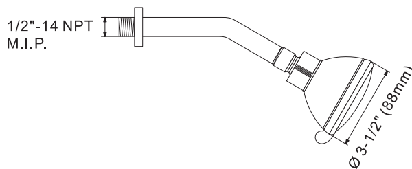
Shower arm / Bras de douche B-028-1 Shower head / Pomme de douche pluie RP-RS125
