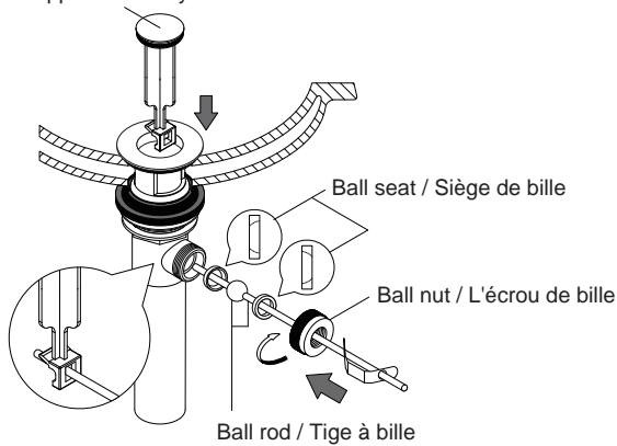
Stopper assembly / Bouchon de la bonde
